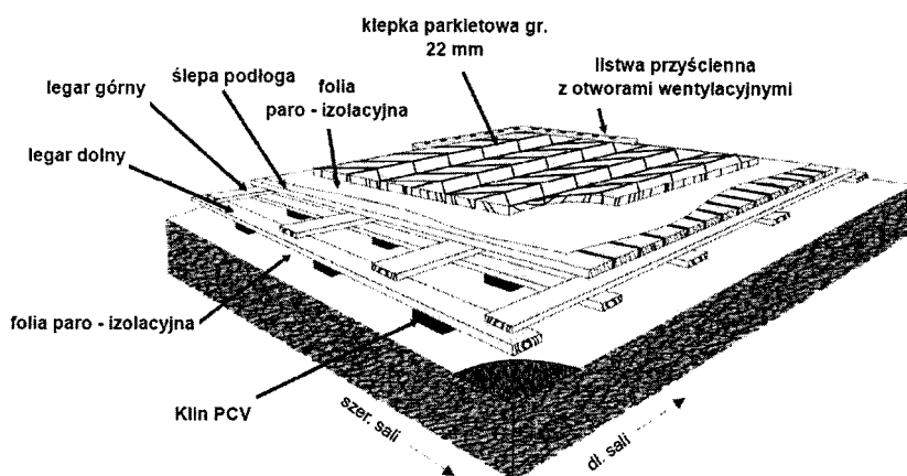
Rys. 1 – Przekrój podłogi sportowej
